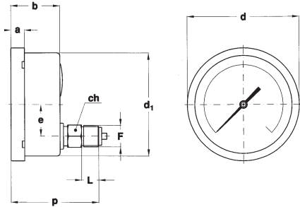
D - Anschluss zentrisch hinten, zur Direktmontage
